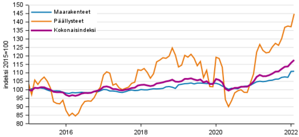
Liitekuvio 1. Maarakennuskustannusindeksi (2015=100), Maanrakennuskustannusindeksi kokonaisindeksi, maarakenteet ja päällysteet, 1/2015–02/2022
